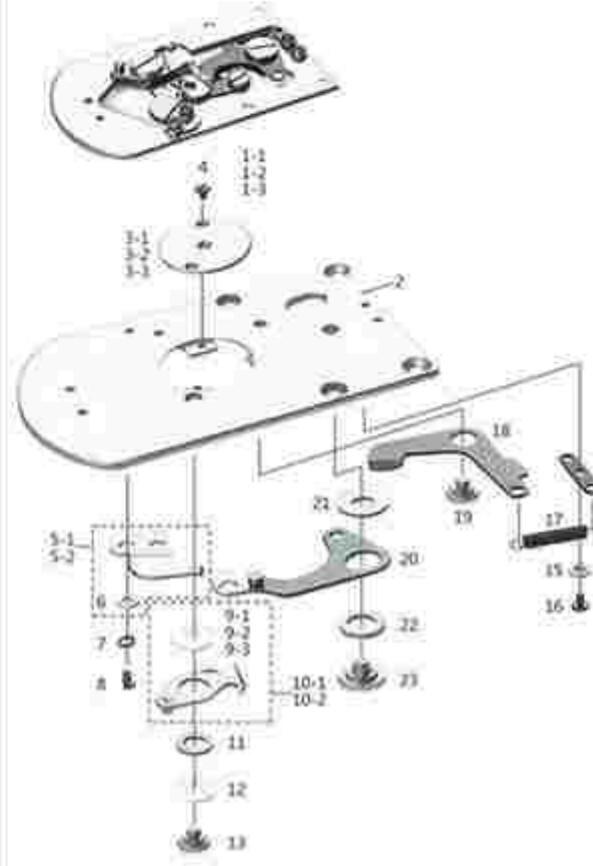
BROTHER/兄弟 KE-430D剪线组件 ASSEMBLY FOR KE-430D
