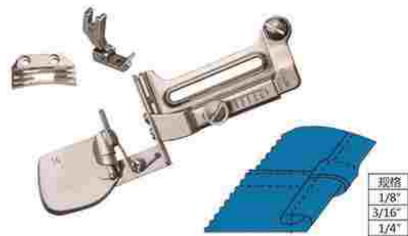
RX-G30 A70/S70 摆动式弹弓咀卷边器 Spring NFpe Swing Hemmer
