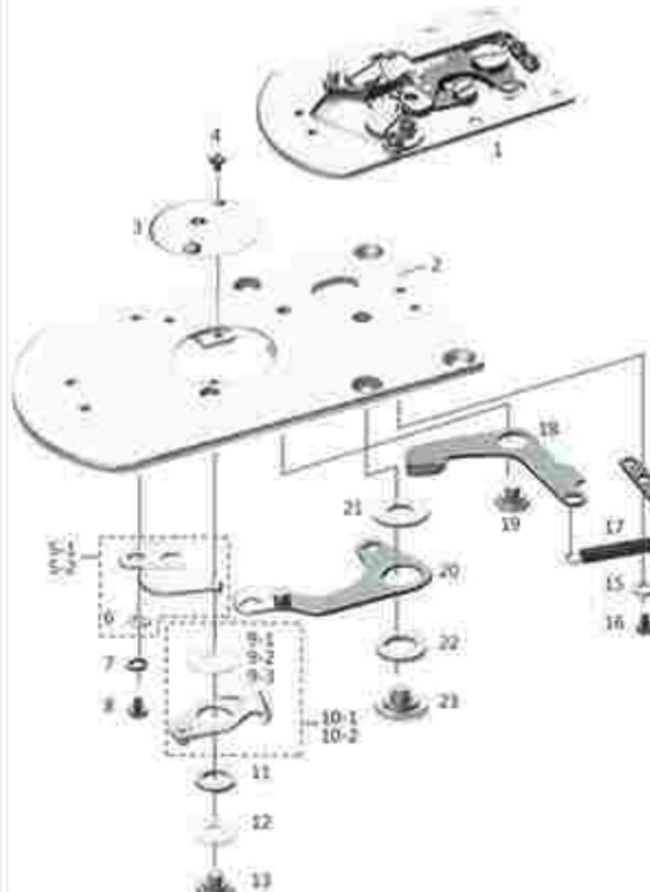
BROTHER/兄弟 BE-438D剪线组件 ASSEMBLY FOR BE-438D
