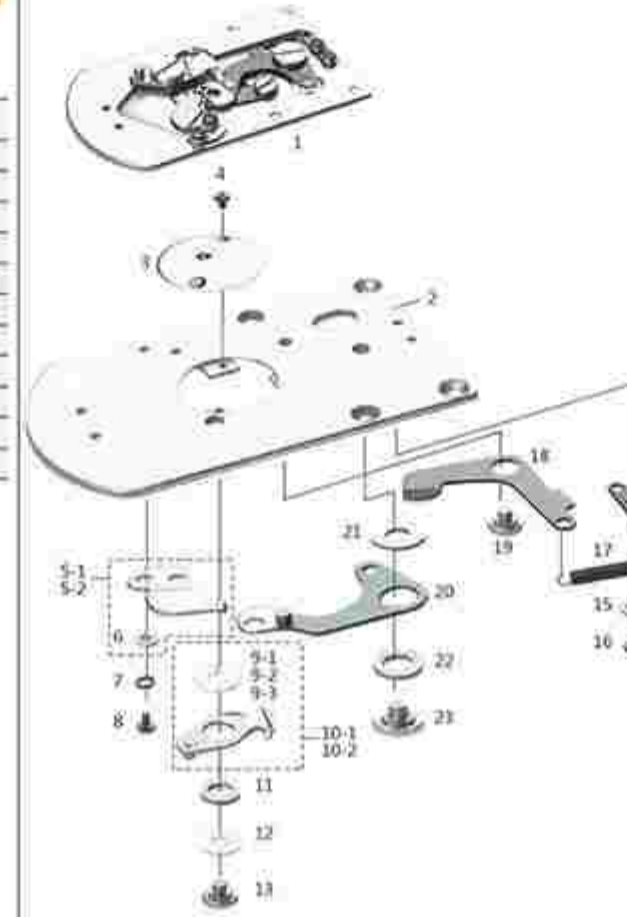
BROTHER/兄弟 KE-430E剪线组件 ASSEMBLY FOR KE-430E
